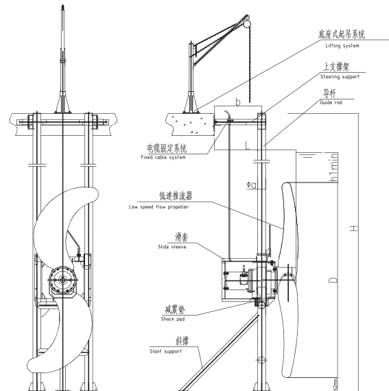
VII型安装
