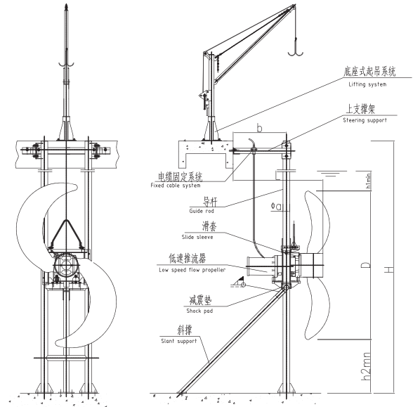
V型安装
