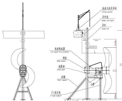
VI型安装
