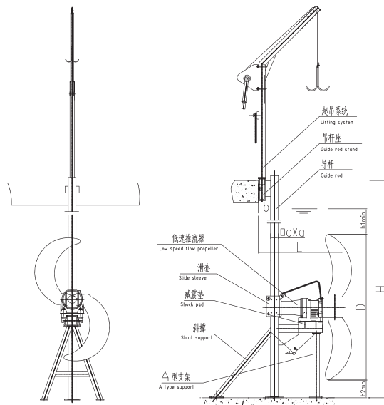
IV型安装
