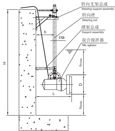
I型安装
