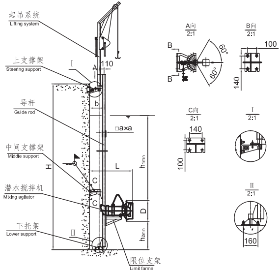
II型安装
